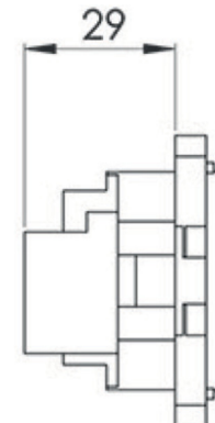
SIDE (LID)
